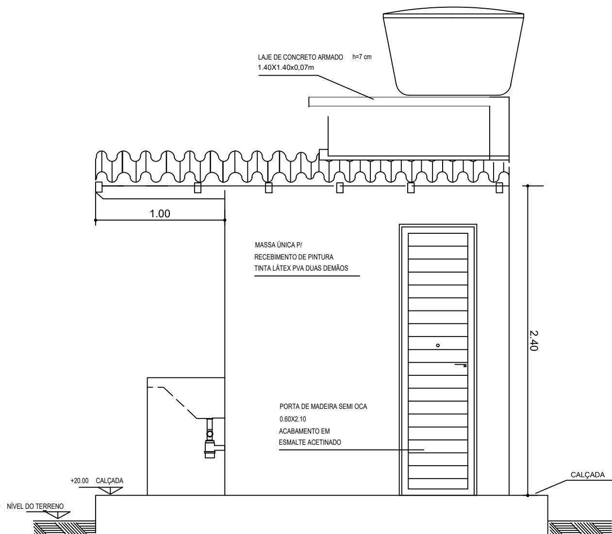
VISTA LATERAL ESC: 1:25
