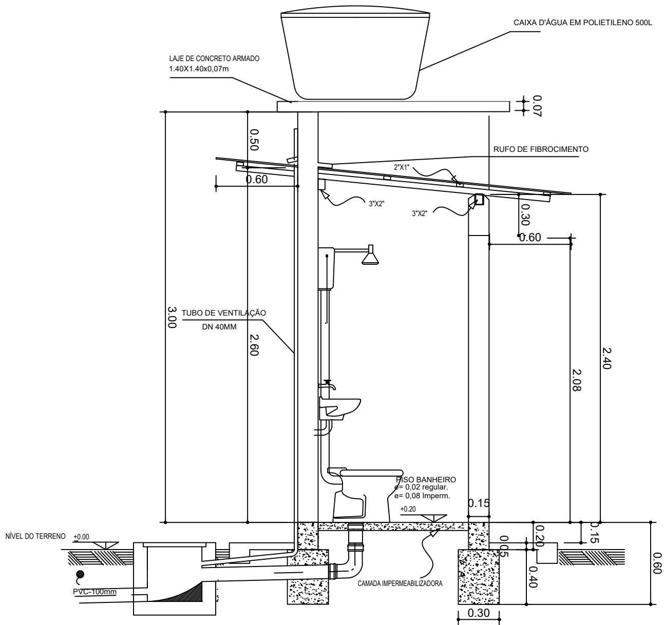
CORTE AB ESC: 1:25
